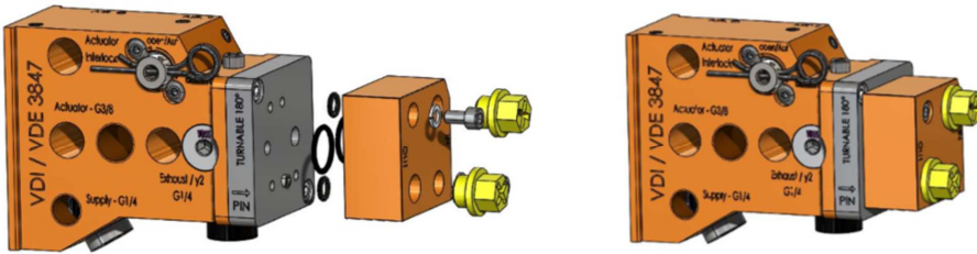
Abb. 73 Anschlussplatte für Magnetventil AP-1107.
